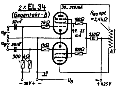
Schaltung 5. Praktisches Schaltbeispiel für Gegentakt-B-Schaltung mit fester Gittervorspannung und 425 V Betriebsspannung (Einstellung nach Kennlinienfeld 9).
