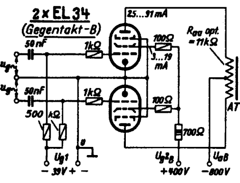
Schaltung 7. Praktisches Schaltbeispiel für Gegentakt-B-Schaltung mit fester Gittervorspannung und voller Ausnützung aller Grenzwerte. Anodenspeisespannung 800 V, Schirmgitterspeisespannung 400 V (Einstellung nach Kennlinienfeld 11).
