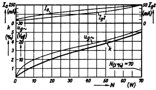
Kennlinienfeld 11 Aussteuerkurven für Gegentakt-B-Schaltung mit maximaler Ausnützung aller Grenzwerte, gemessen mit festen Speisespannungen U_{aB} = 800 V , U_{g2B} = 400 V und fester Gittervorspannung U_{g1} = -39 V , R_{g2} = 750 \Omega , R_{aa} = 11 k\Omega \cdot k , u_{g\sim} und I_a, I_{g2} (für beide Röhren) sowie Anodenverlustleistung Q_a (max. 27,5 W) = f(N) .
