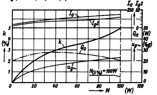
Kennlinienfeld 11 Aussteuerkurven für Gegentakt-B-Schaltung mit maximaler Ausnützung aller Grenzwerte, gemessen mit festen Speisespannungen U_{aB} = 800 V , U_{g2B} = 400 V und fester Gittervorspannung U_{g1} = -39 V , R_{g2} = 750 \Omega , R_{aa} = 11 k\Omega \cdot k , u_{g\sim} und I_a, I_{g2} (für beide Röhren) sowie Anodenverlustleistung Q_a (max. 27,5 W) = f(N) .
