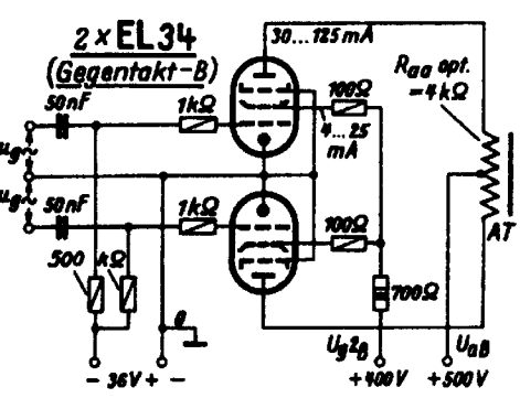
Schaltung 6. Praktisches Schaltbeispiel für Gegentakt-B-Schaltung mit fester Gittervorspannung und 500 V Anodenspeisespannung bzw. 400 V Schirmgitterspeisespannung (Einstellung nach Kennlinienfeld 10).
