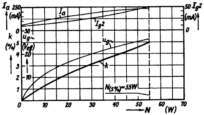
Kennlinienfeld 9 Aussteuerkurven für Gegentakt-B-Schaltung mit fester Vorspannung ( U_{g1} = -38 V ), gemessen mit U_B = 425 V (fest), R_{g2} = 1 k\Omega , R_{aa} = 3,4 k\Omega \cdot k , u_{g\sim} und I_a, I_{g2} (für beide Röhren) = f(N) .
